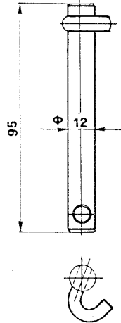
SE 187 PERNO SUPERIORE
