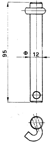
SE 101 PERNO SUPERIORE
